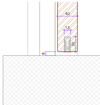
coupe bas porte affleurée cadre 3 pc affleuré
