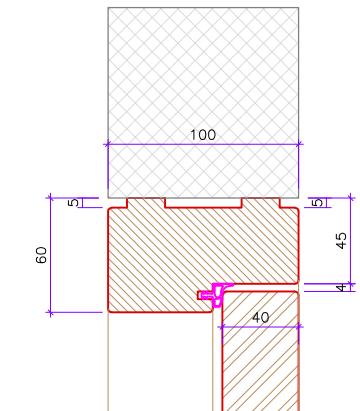
coupe haut porte affleurée cadre bloc affleuré
