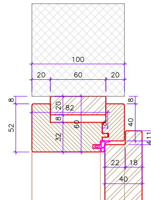
coupe haut porte cadre 2 pc affleuré
