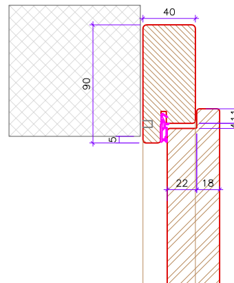
coupe haut porte cadre
