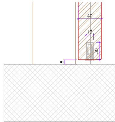
coupe bas porte cadre 2 pc affleuré
