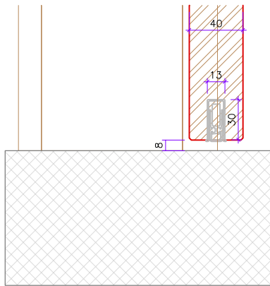
coupe bas porte cadre fx-c. embr.
