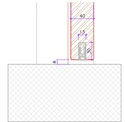
coupe bas porte affleurée cadre bloc affleuré
