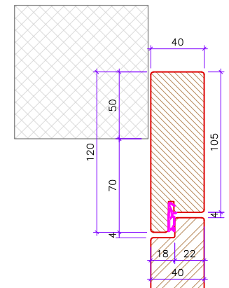
coupe haut porte cadre affleuré
