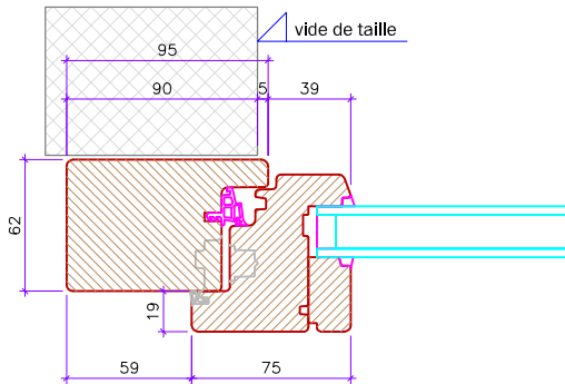
plan côté fenêtre
