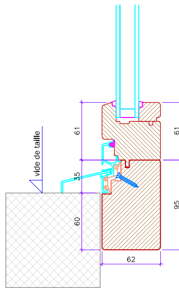
coupe bas fenêtre fixe
