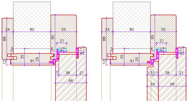
coupe haut palière cadre fx-c. embr. coupe haut palière cadre fx-c. embr.
