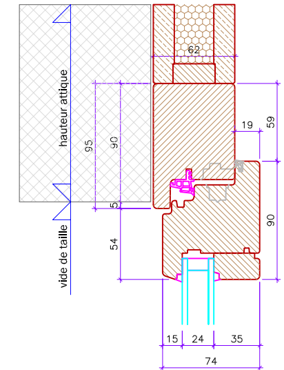
coupe haut porte-fenêtre
