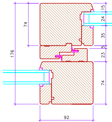
plan milieu fenêtre coulissante
