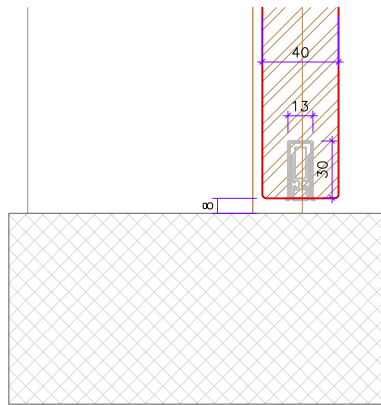
coupe bas porte cadre 2 pc
