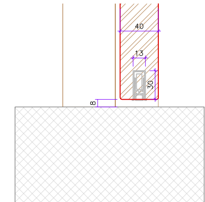
coupe bas porte affleurée cadre 2 pc affleuré
