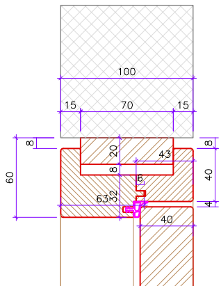
coupe haut porte affleurée cadre 2 pc affleuré
