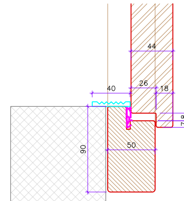
coupe bas porte cadre ei
