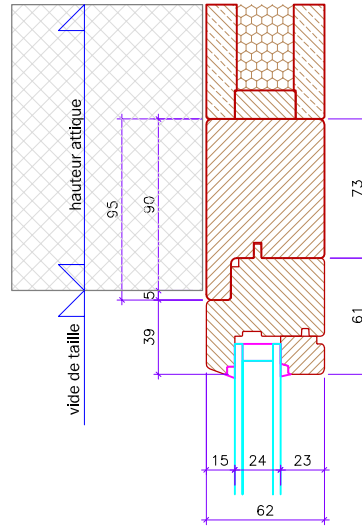
coupe haut fenêtre fixe
