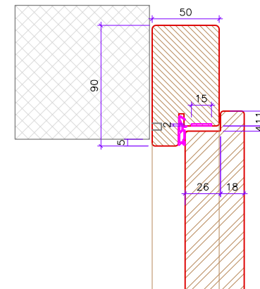
coupe haut porte cadre ei
