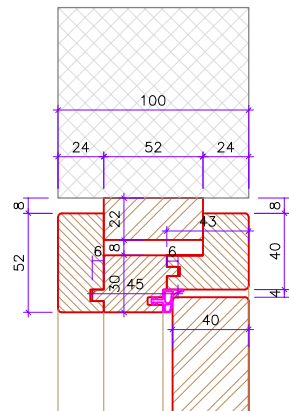
coupe haut porte affleurée cadre 3 pc affleuré
