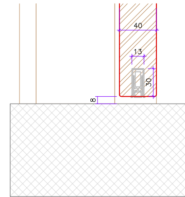
coupe bas porte affleurée cadre fx-c. embr.
