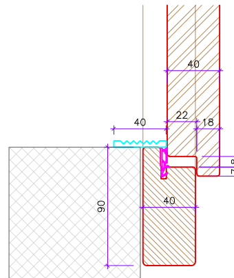
coupe bas porte cadre
