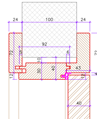
coupe haut porte affleurée cadre fx-c. embr.
