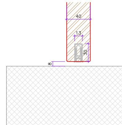
coupe bas porte cadre affleuré
