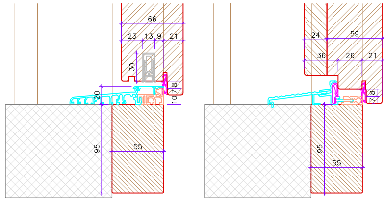
coupe bas palière cadre fx-c. embr. coupe bas palière cadre fx-c. embr.
