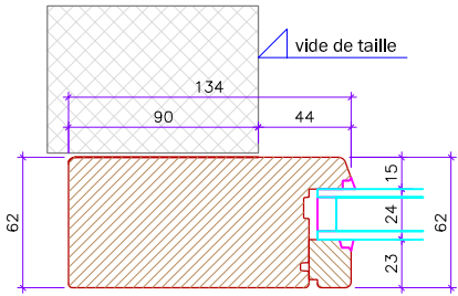
plan côté fenêtre fixe
