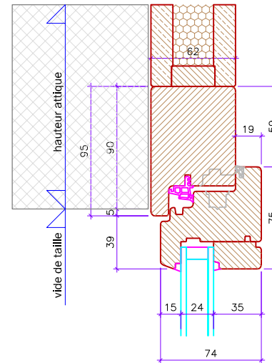
coupe haut fenêtre
