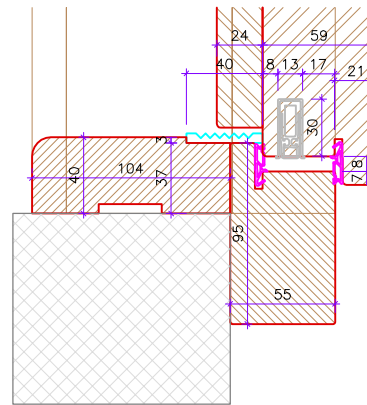
coupe bas palière cadre fx-c. embr.
